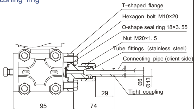
F1/F2 flushing ring
